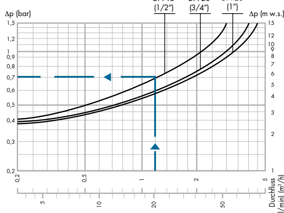
Diagramm 2 (Druckabfall)
